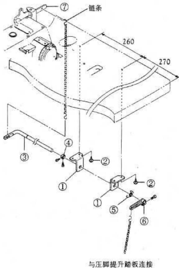
踏板安装到台板左侧时
