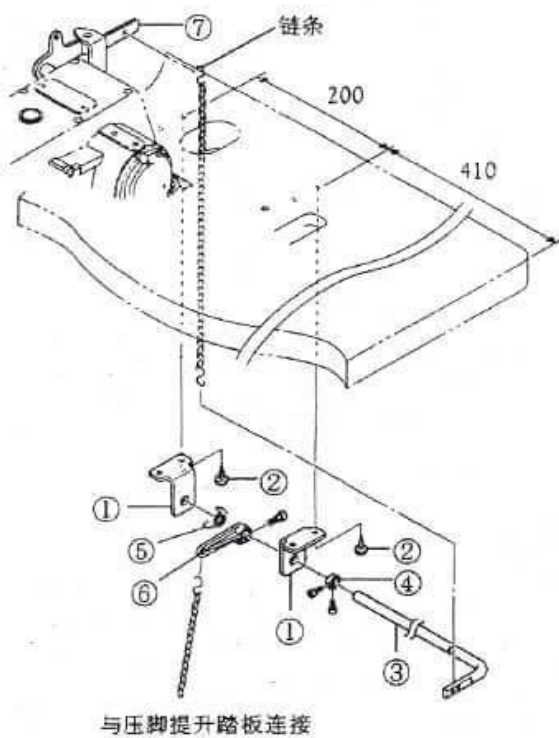
踏板安装到台板右侧时
